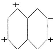
D.R.P. 22038. Höchstler Farbwerke.
